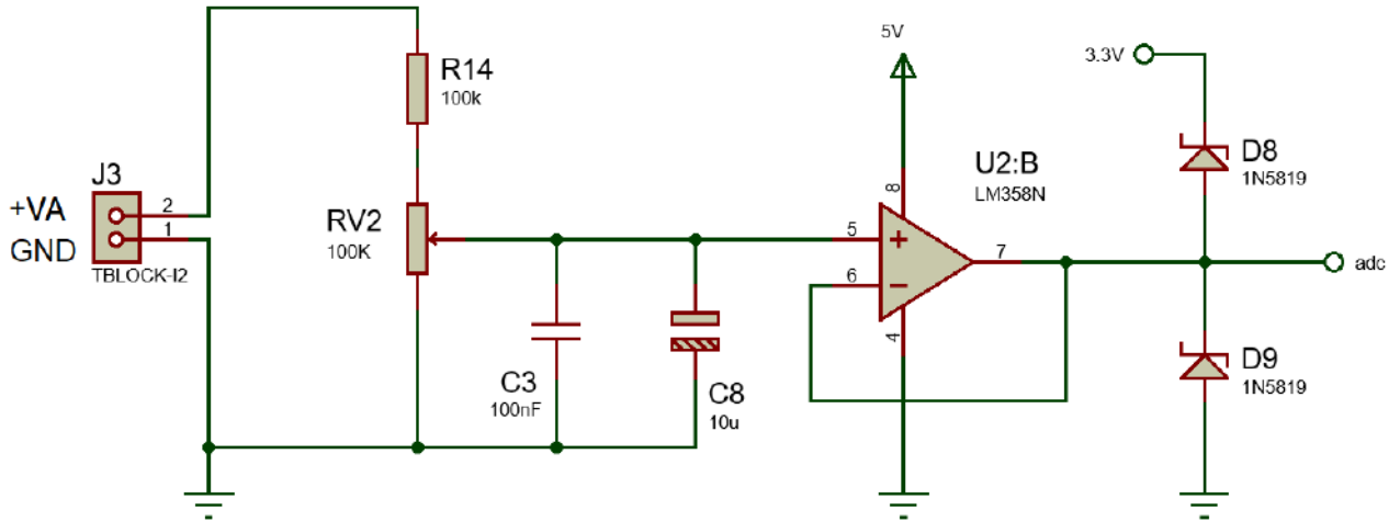
Fig 3. Circuito para la entrada analógica ( 0 V \leq V_A \leq 10 V ).
