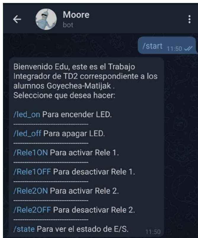
Fig 8. Captura de pantalla del chat con el bot.
