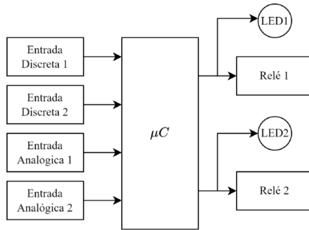
Fig 1. Diagrama de bloques del circuito.
