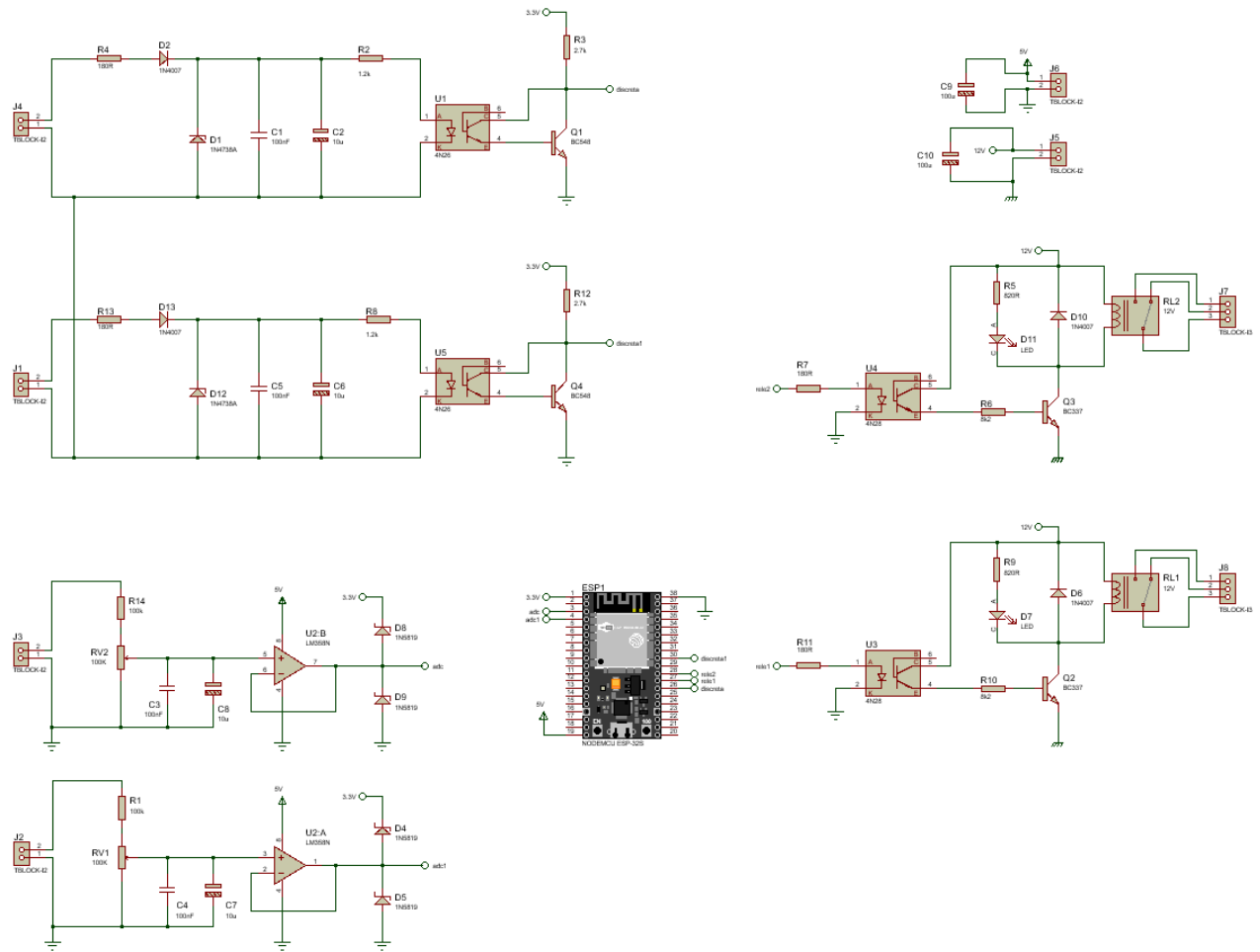
Fig 5. Esquema del circuito.
