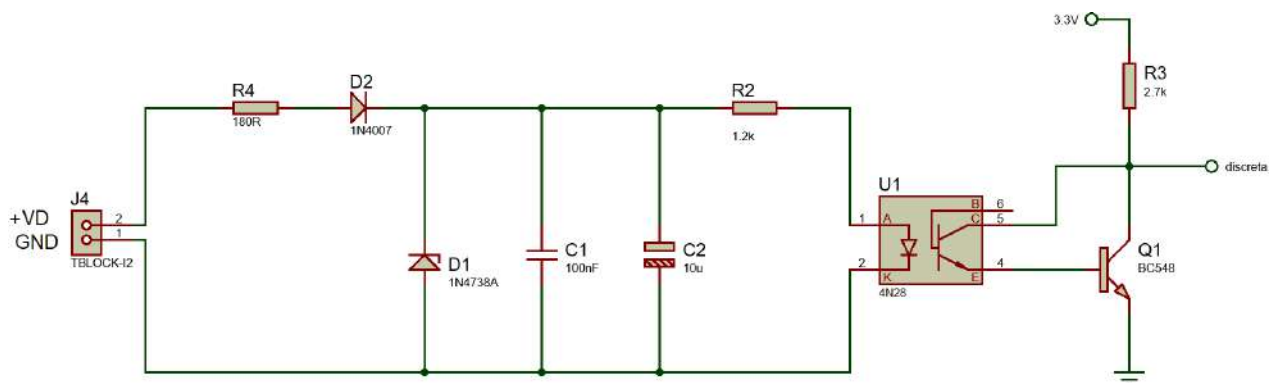
Fig 2. Circuito para la entrada discreta ( 10\text{ V} \leq V_D \leq 25\text{ V} ).
