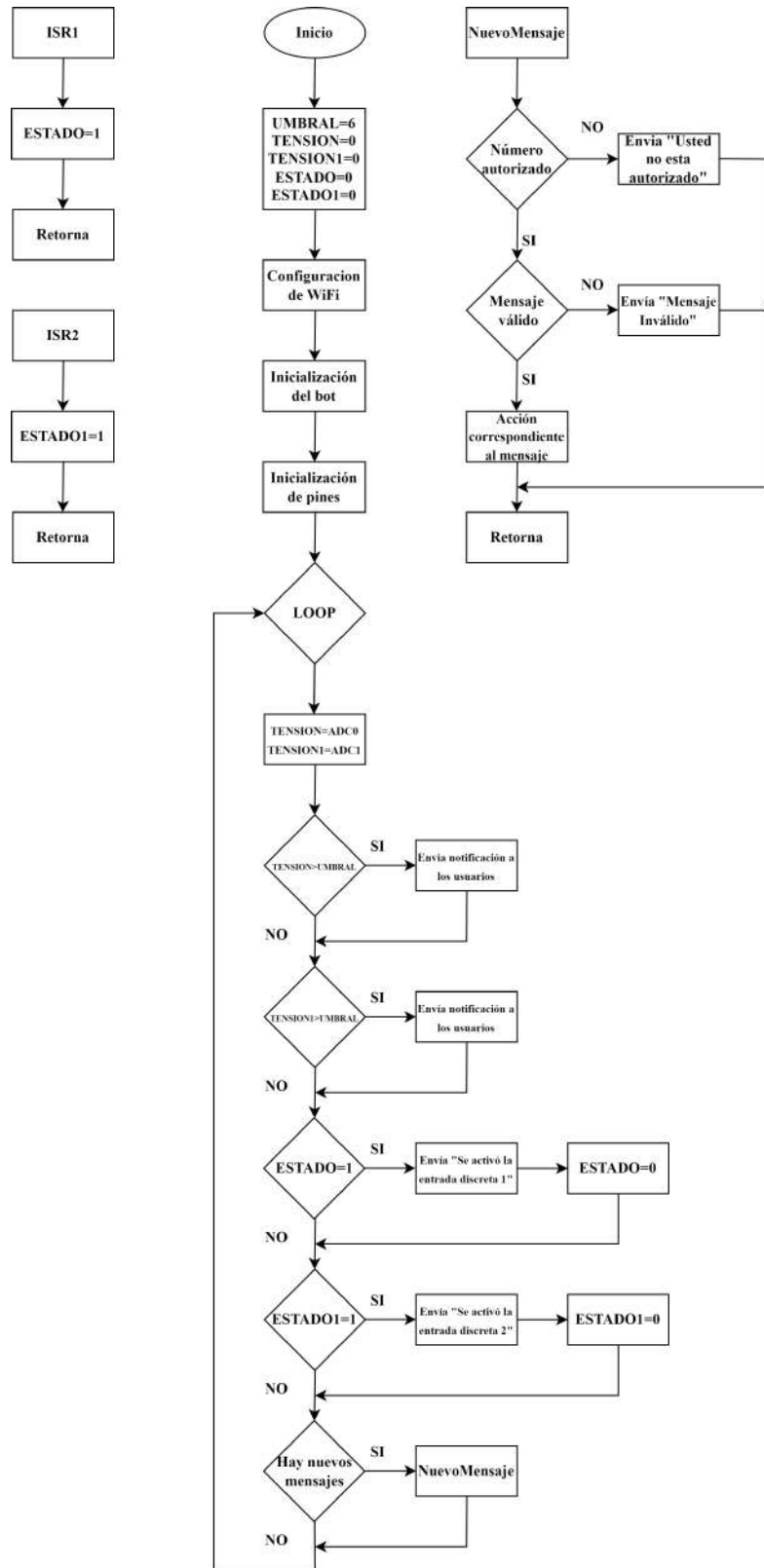
Fig 7. Diagrama de flujo del programa.
