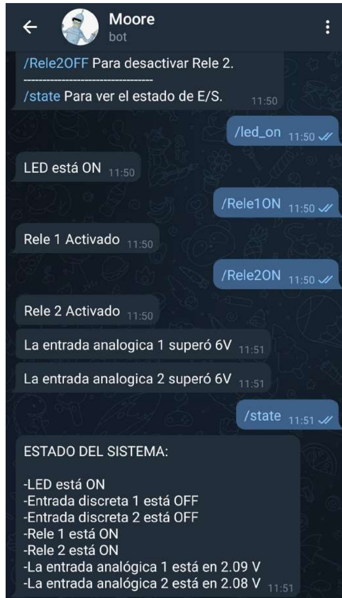
Fig 9. Captura de pantalla del chat con el bot con diferentes instrucciones.
