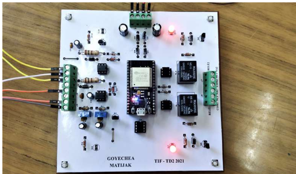
Fig 12. Circuito final en funcionamiento.
