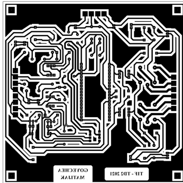
Fig 10. PCB del sistema diseñado.
