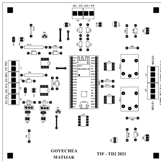
Fig 11. Máscara de componentes (Top Silk).
