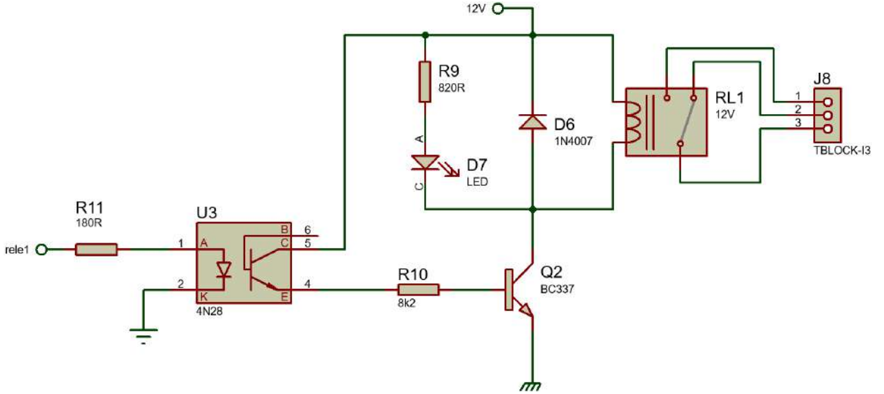
Fig 4. Circuito de salida.
