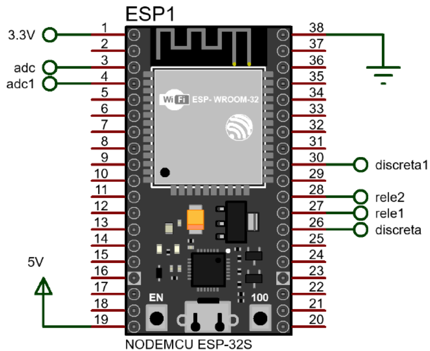
Fig 6. Conexiones al ESP32.
