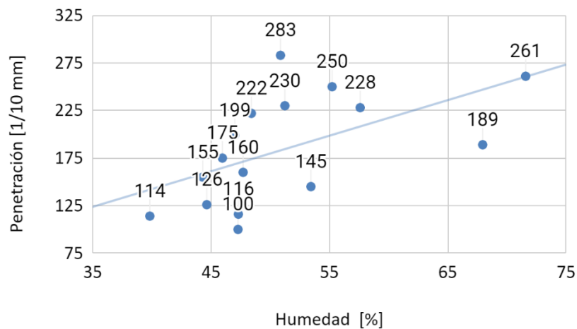
Fig. 15. LP-Valores de Penetración-Humedad en suelo seco para porcentajes de cemento 2, 4, 6, 8%.
