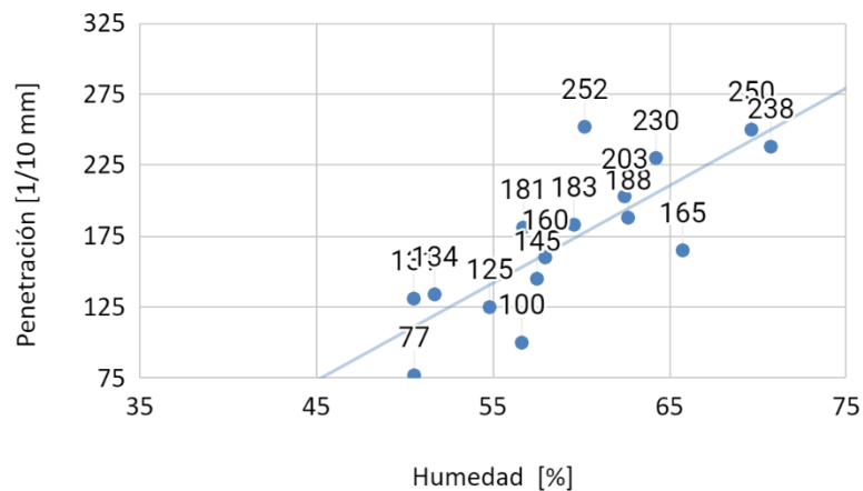
Fig. 16. LL-Valores de Penetración-Humedad en suelo secado a aire para porcentajes de cemento 2, 4, 6, 8%.
