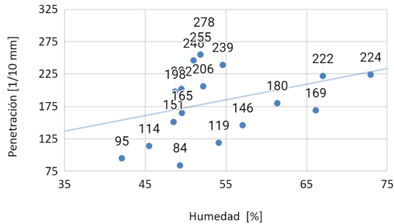
Fig. 14. LL-Valores de Penetración-Humedad en suelo seco para porcentajes de cemento 2, 4, 6, 8%.
