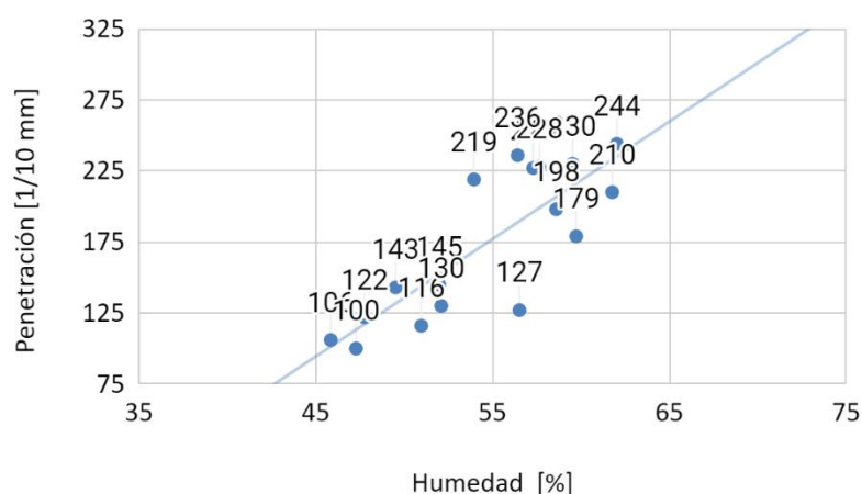
Fig. 17. LL-Valores de Penetración-Humedad en suelo secado a aire para porcentajes de cemento 2, 4, 6, 8%.
