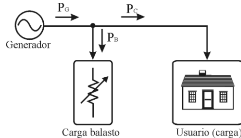
Figura 15. Sistema de regulación por carga balasto.
