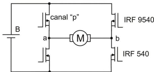
Figura 12. Etapa de potencia en puente H completo, con MOSFET de canal P y N .
