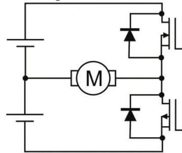
Figura 10. Comando de potencia con utilizando transistores MOS-FET.
