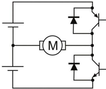
Figura 9. Comando de potencia con utilizando transistores BJT.
