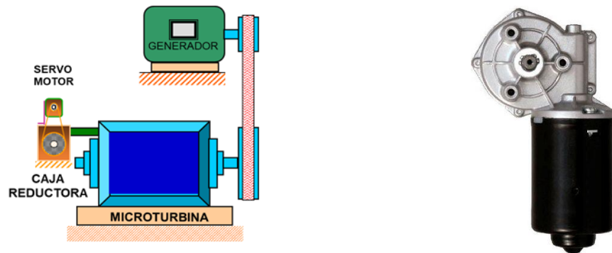
Figura 4. Croquis del grupo turbogenerador e imagen de un tipo de motor de accionamiento utilizado. Fuente: elaboración propia
