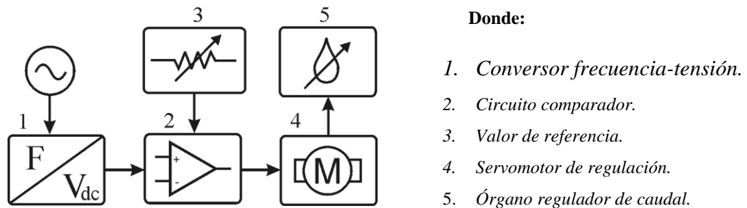
Figura 3. Regulador de frecuencia por variación de caudal
