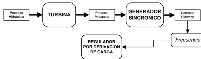
Figura 16. Regulación de frecuencia por carga balasto.
