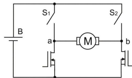
Figura 13. Etapa de potencia en puente H híbrido
