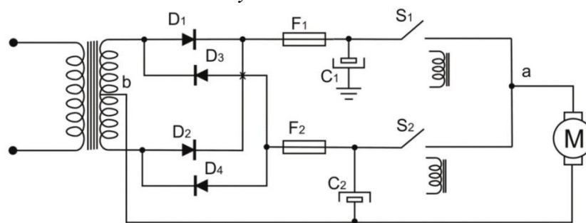
Figura 7. Comando de motor con relés electromecánicos. Fuente: elaboración propia
