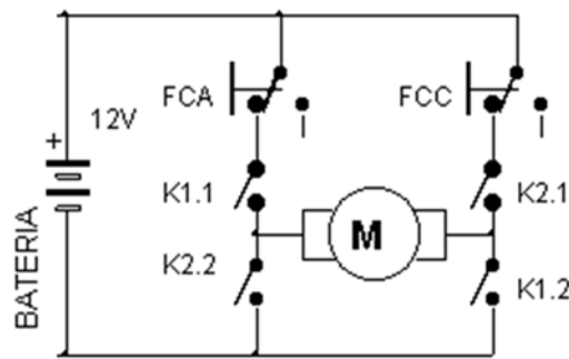
Figura 11. Puente H conformado por cuatro llaves electromecánica (relés).
