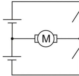
Figura 8. Esquema básico, con fuente simétrica.
