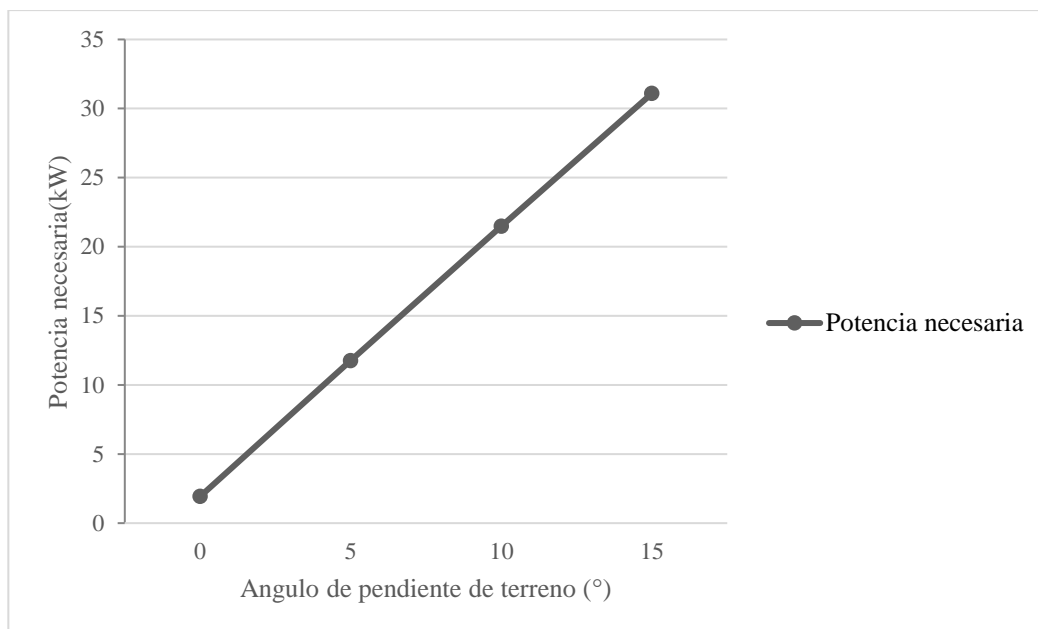
Fig. 2. Potencia necesaria a 50 km/h con motor 4 kW y conjunto de baterías de mínimo peso.
