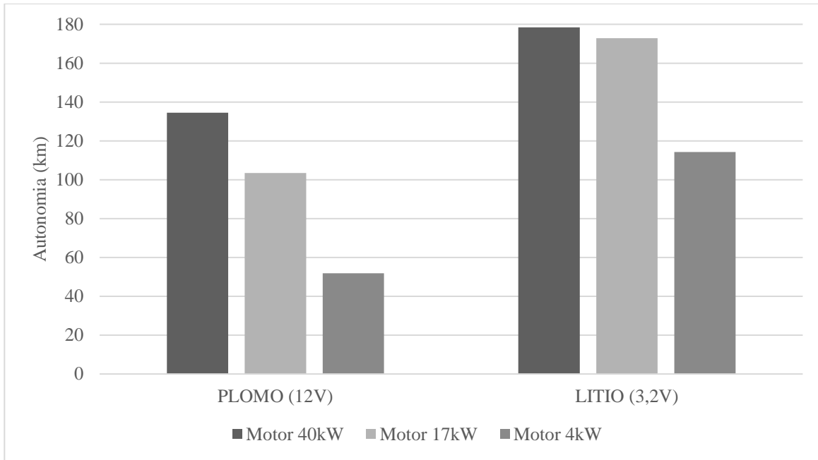
Fig. 1. Comparación de distintas autonomías de conjunto de baterías y motores.
