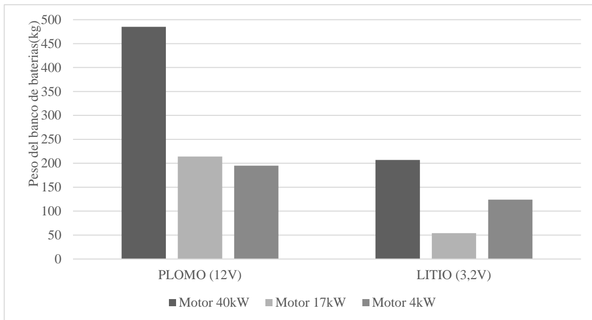
Fig. 1. Comparación de peso de conjunto de baterías y motores.
