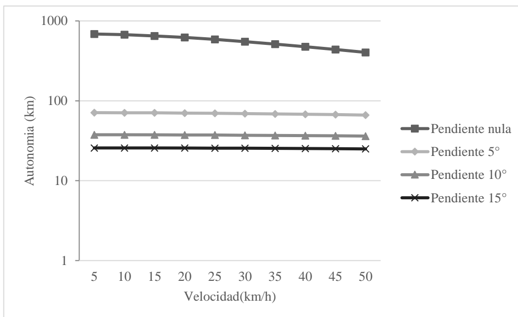
Fig. 4. Autonomía teórica conjunto motor 17 kW y baterías de litio para distintas velocidades/pendientes de terreno.
