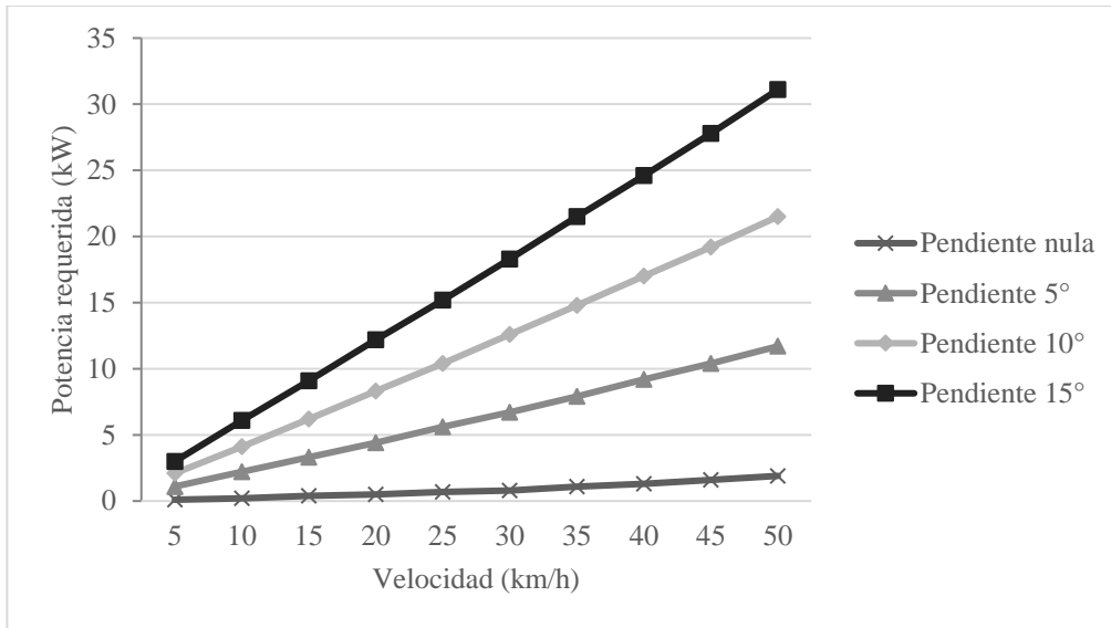
Fig. 3. Potencia requerida para distintas pendientes de terreno con motor de 17 kW y baterías de litio.
