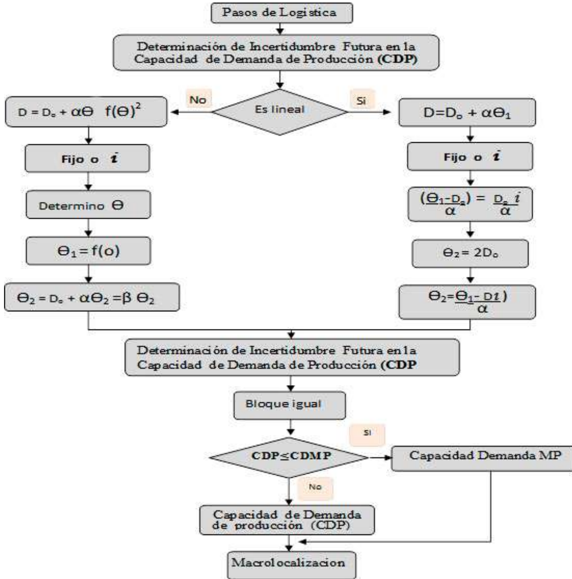
Figura 3. Procedimiento específico para la definición del tamaño inicial de la instalación y su macro localización. Fuente: Elaboración propia (2016).
