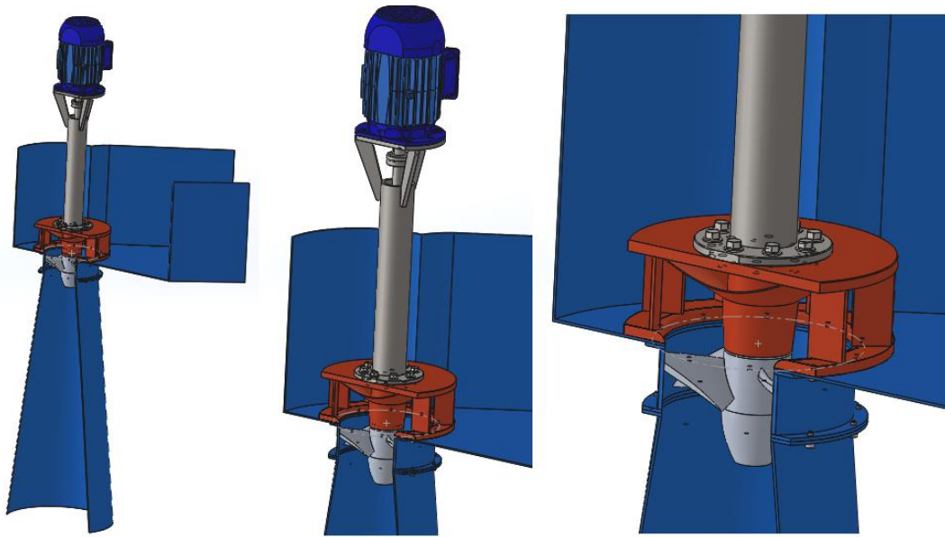
Figura 2- Conjunto de picogeneración completo (detalles de izq. a der.)
