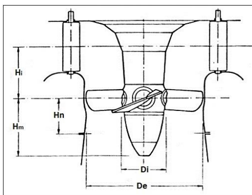
Figura 1- Dimensiones generales turbina hidráulica axial .
