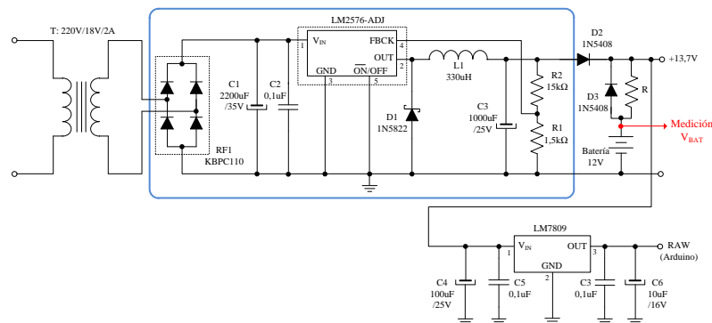
Figura 4: Fuente de tensión conmutada tipo Buck.
