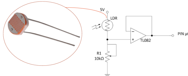
Figura 3: LDR con su etapa de acondicionamiento de la señal.
