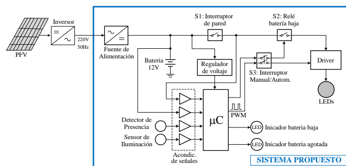
Figura 1: Diagrama en bloques del sistema de iluminación LED.
