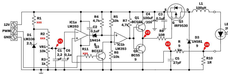
Figura 2: Esquema eléctrico del driver de la lámpara LED.
